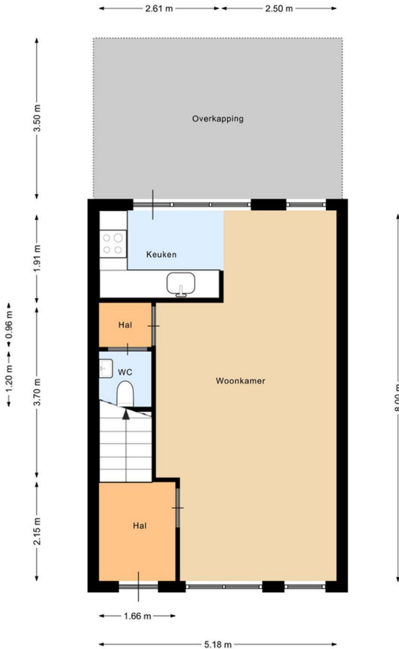
Begane Grond
