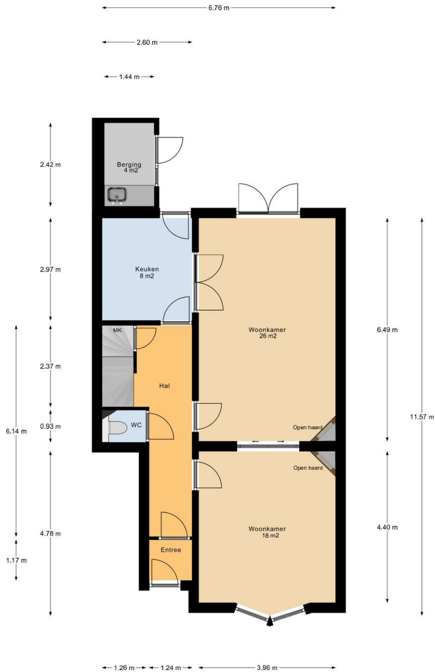
Begane Grond
