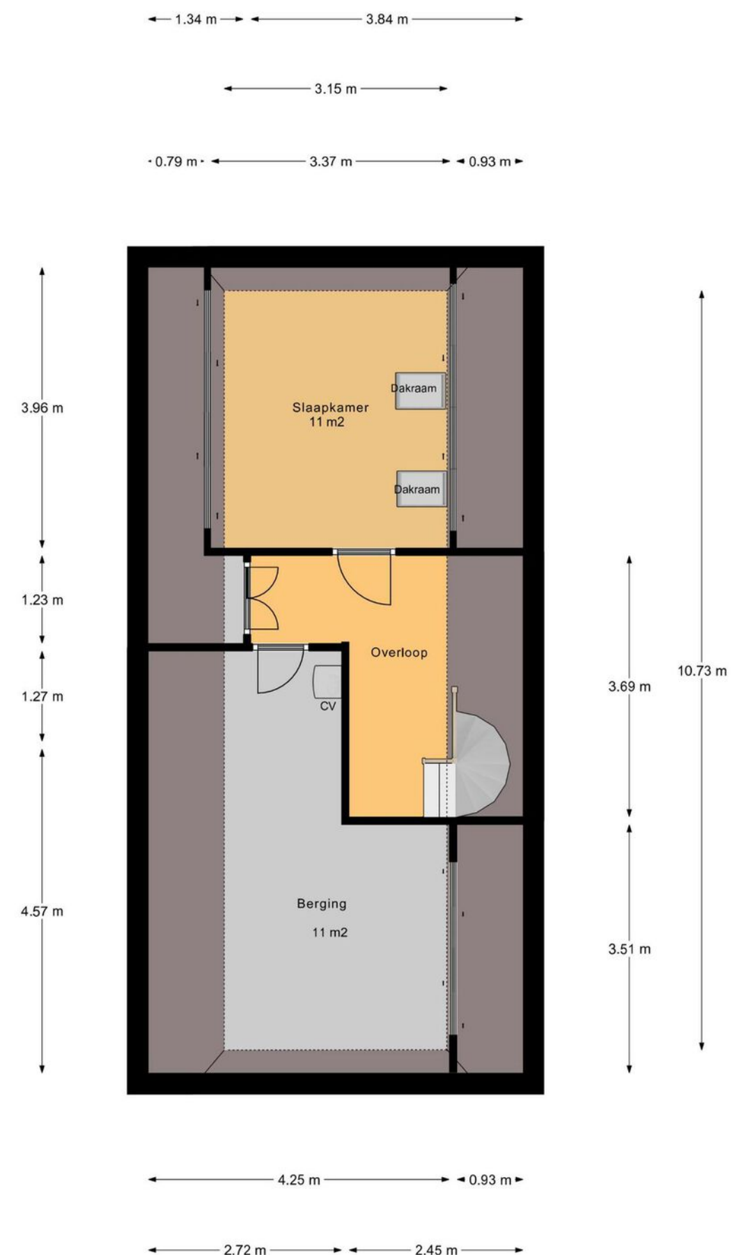
2e Verdieping
